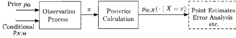
图 5: 贝叶斯推断模型
